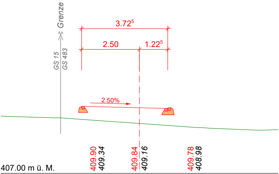
QP Nr. 1 km 10.0
