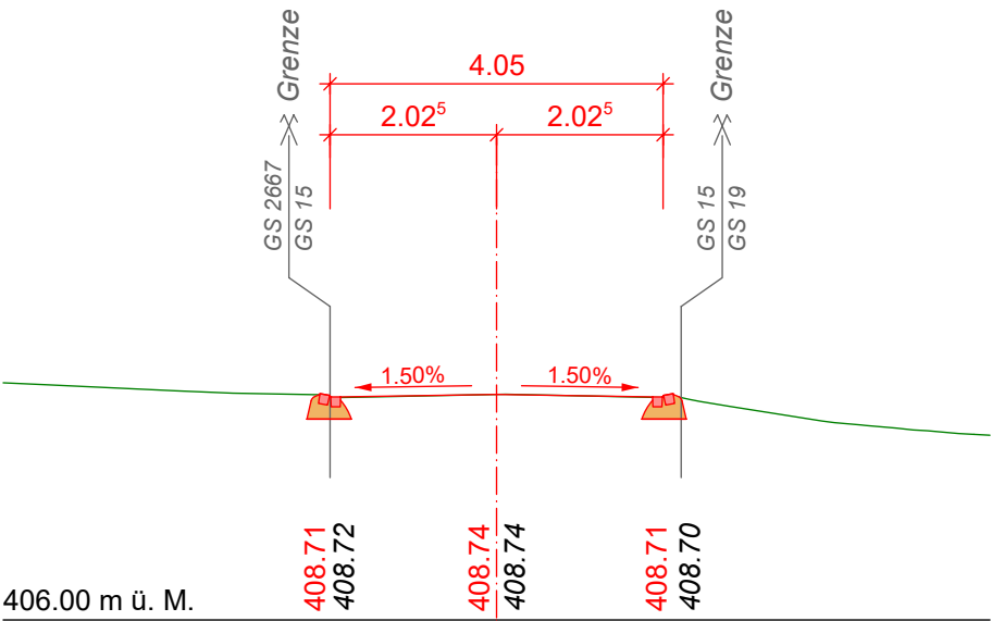
QP Nr. 4 km 34.11
