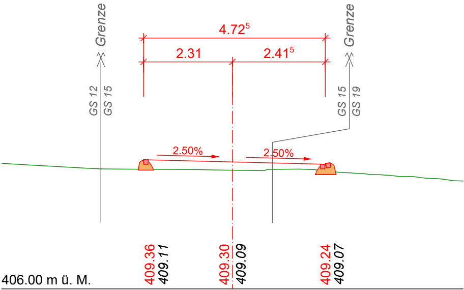
QP Nr. 2 km 20.00
