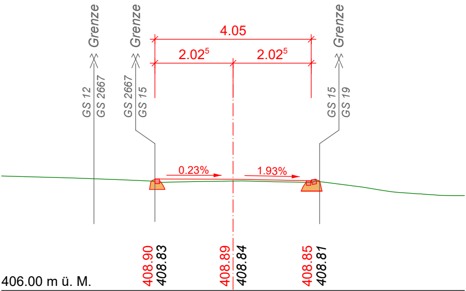
QP Nr. 3 km 30.00
